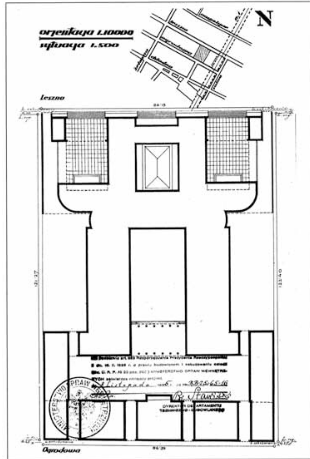
77. Projekt realizacyjny Sądu Grodzkiego, orientacja i sytuacja, 1935, AAN MSW 3643
