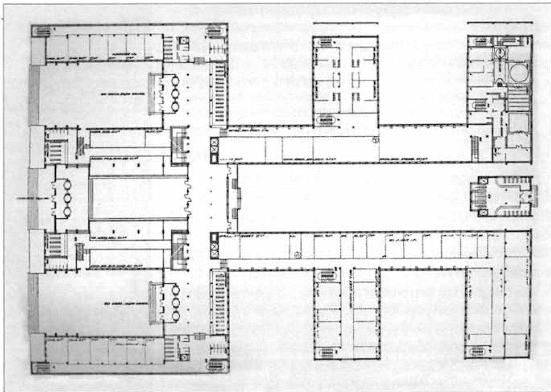
B. Pniewski, projekt konkursowy gmachu sądów grodzkich w al. Solidarności 127, 1935 Poprzeczny układ głównego holu równoważy podłużną oś gmachu
